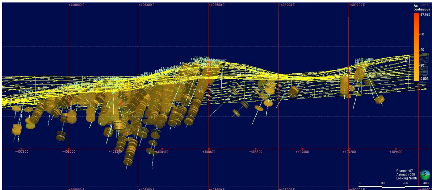
Diagram 2. Fran Gold Au >0.1 g/t cutoff
